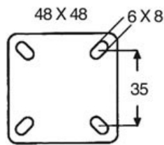
PIASTRE - PLATES
