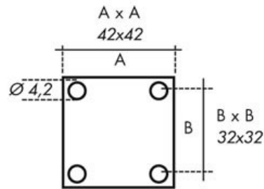
PIASTRE - PLATES
